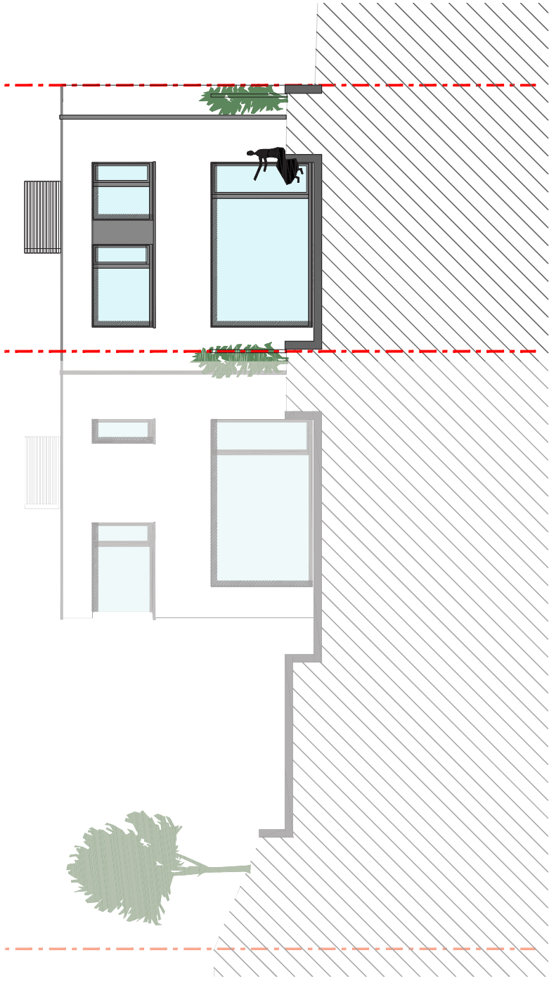
élévation arrière
